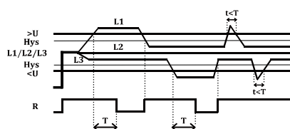
过压、欠压监控功能图
