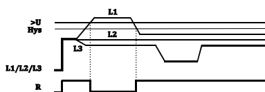
过压监控功能图
